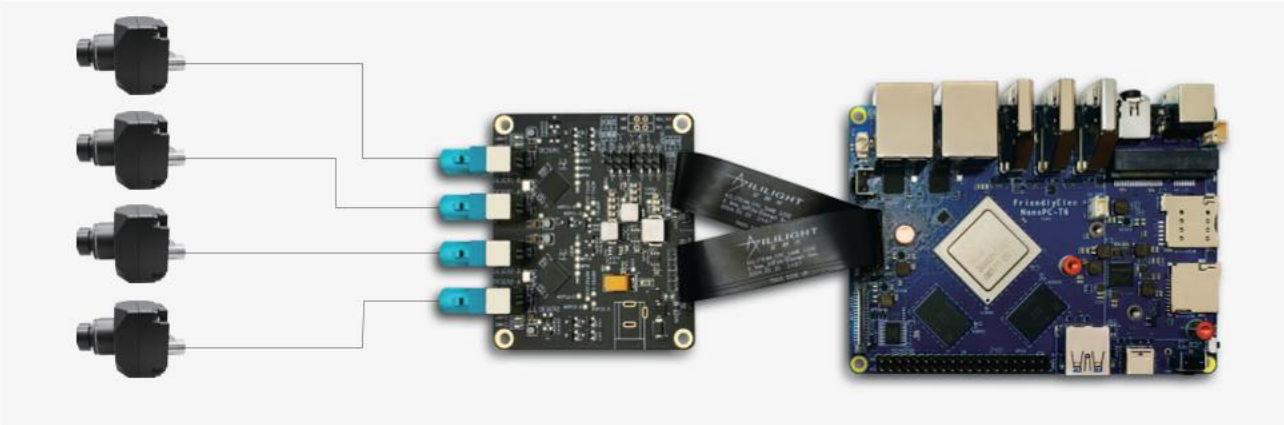
3M摄像头模组*4 GMSL转接套件 瑞芯微RK3588开发板
